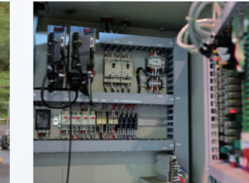
配電盤
